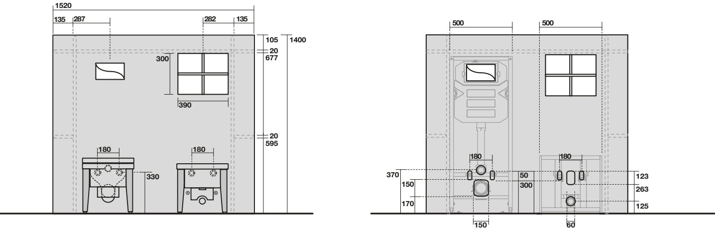
9184 Mobile pannello in legno 90x140x17 completo di struttura per wc sospeso e cassetta di scarico priva di placca Wooden unit 90x140x17 depth w/concealed cistern without flushing plate and metal brackets for wall hung wc
