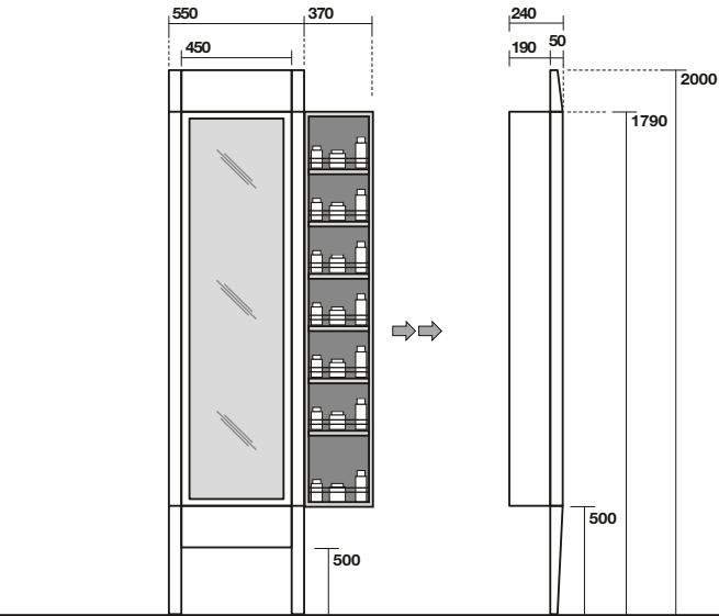
9183 Specchio a terra con contenitore estraibile 55x200x24 Mirror cabinet w/hideaway shelves 55x200x24
